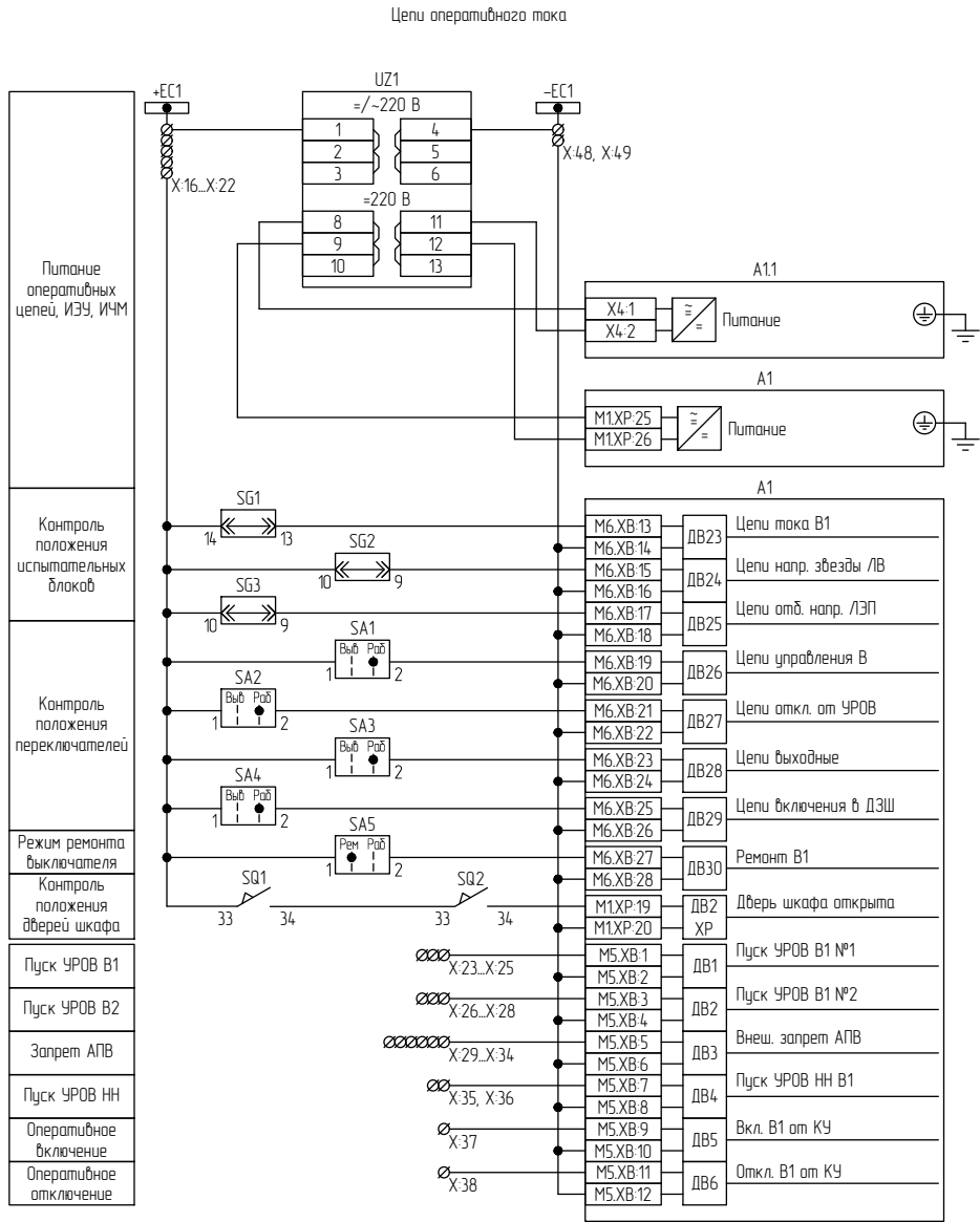
Рисунок В.2 – Схема электрическая принципиальная (часть 2)
