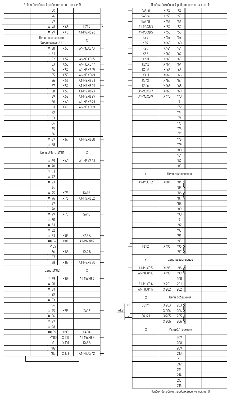
Рисунок Г.2 – Схема электрическая соединений рядов зажимов (часть 2)
