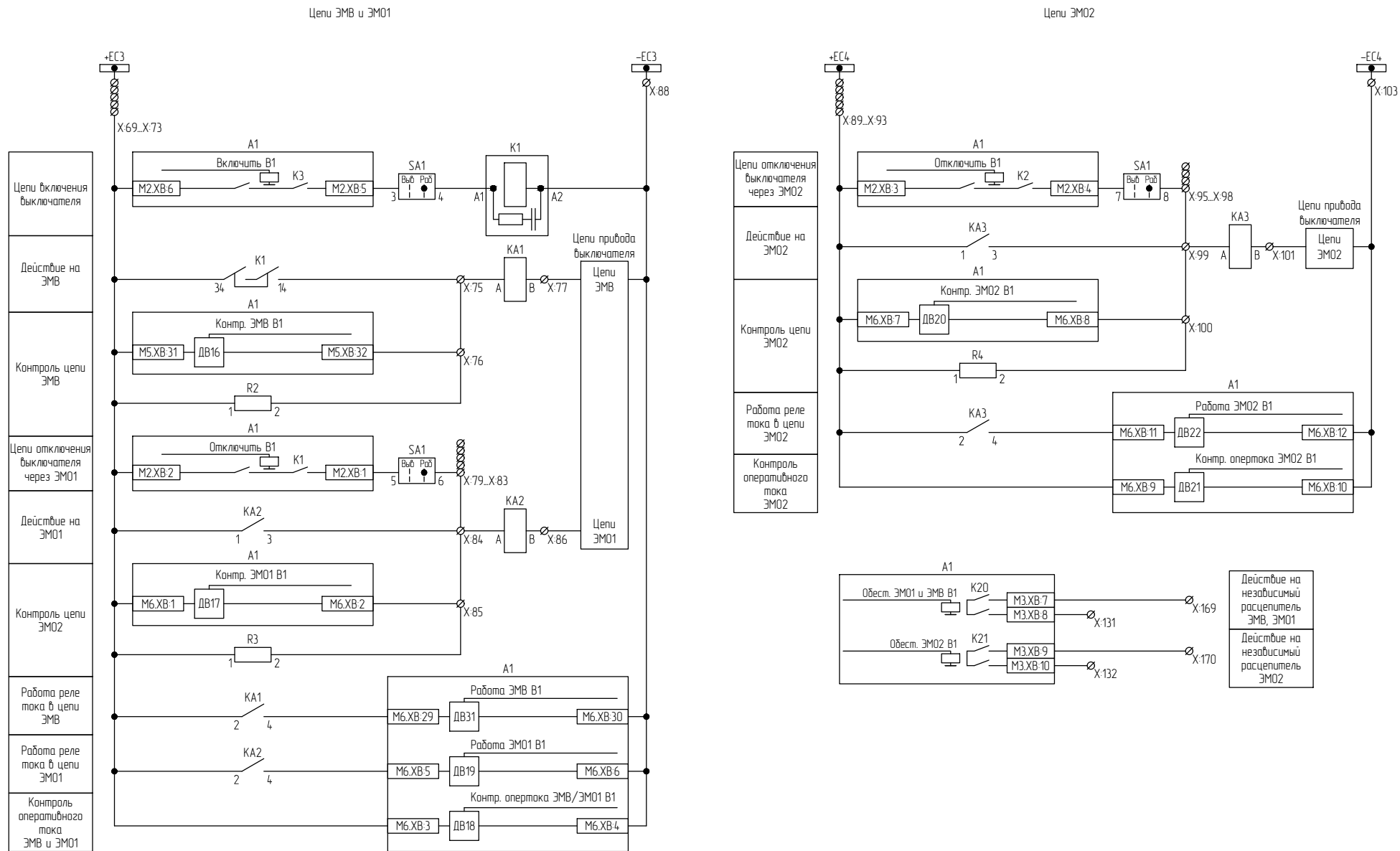
Рисунок В.3 – Схема электрическая принципиальная (часть 3)
