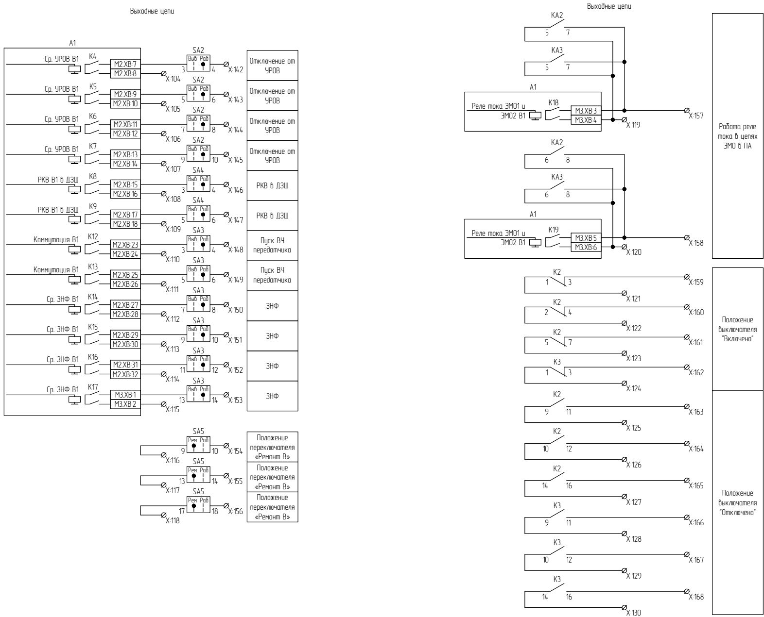
Рисунок В.4 – Схема электрическая принципиальная (часть 4)
