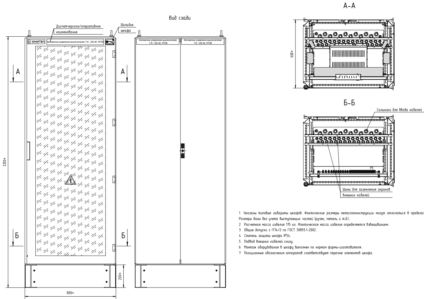
Рисунки Б.1 – Чертеж общего вида (часть 1)
